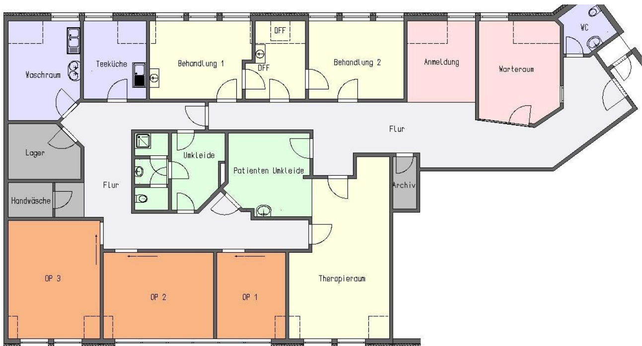
Grundriss
